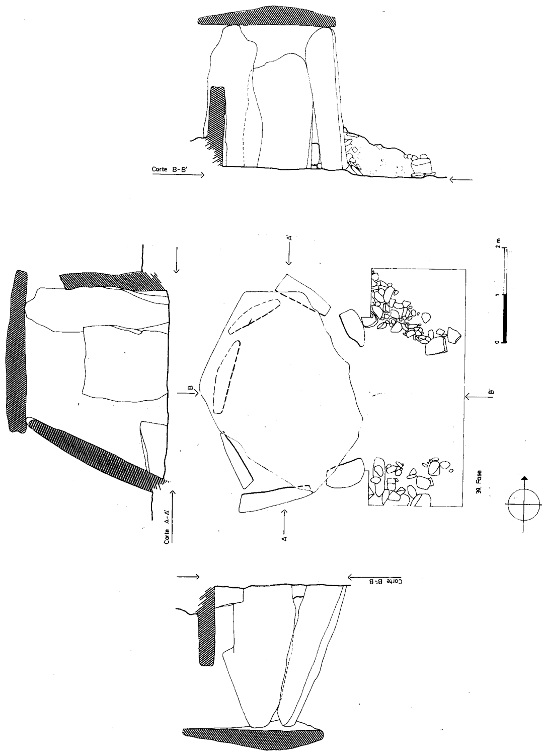
Fig. 6 - Planta e vistas em secção do monumento, após a escavação e antes do restauro. Lev. de J. Luís Madeira e J. Augusto A. Dias. Des. de J. Luís Madeira.
