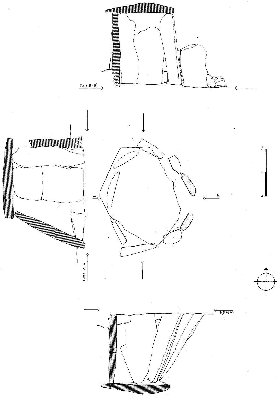
Fig. 7 - Planta e vistas em secção do monumento, após o restauro; a pontilhado indicam-se os esteios que foram recolocados nos prováveis sítios originais. Lev. de J. Luís Madeira e J. Augusto A. Dias Des. de Luís Madeira.
